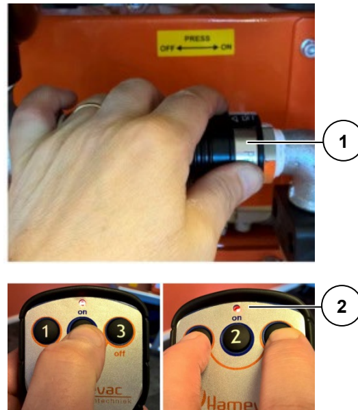
Figure 17 : 8.3.5 Valve manuelle / Télécommande
