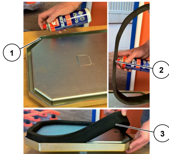
Figure 22 : Mise en place du caoutchouc de la ventouse
