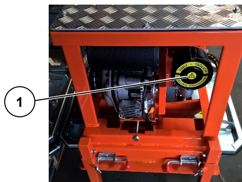
Figure 19 : Contrôle du filtre
