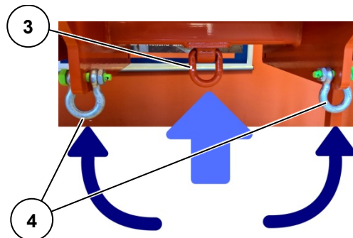
Figure 9 : Fixation à la machine (exemple)
