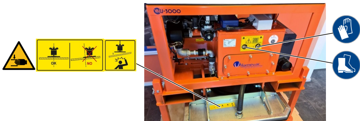
Figure 5 : Emplacements des symboles de sécurité
