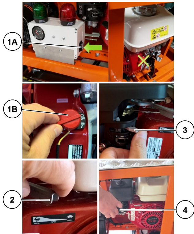
Figure 133 : Mise en marche VHU-3000-B/BVU
