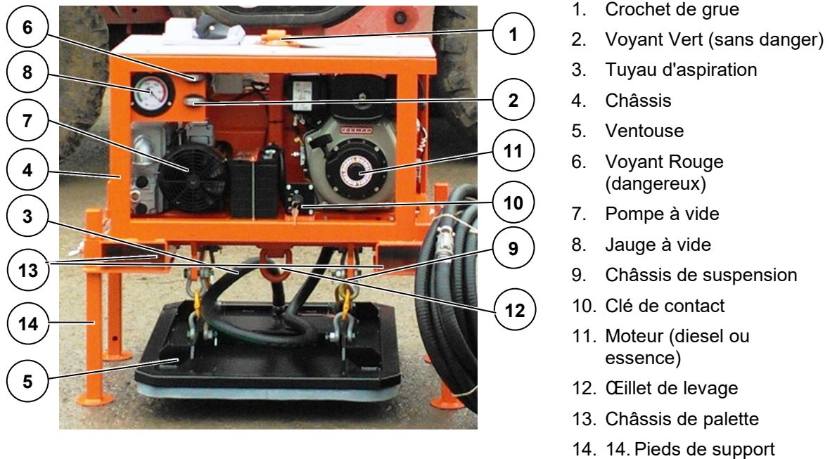
Figure 2 : Composants principaux de la machine
