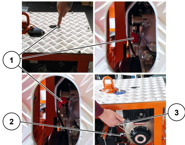
Figure 155 : Mise en marche VHU-3000-D
