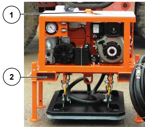
Figure 9 : Fixation à la machine (exemple)
