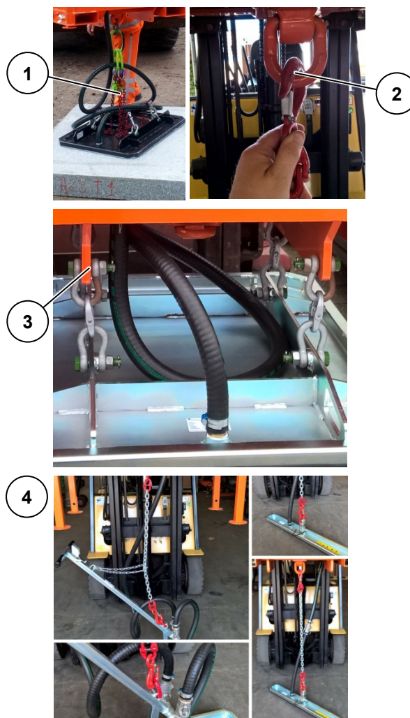
Figure 11 : Suspension d'une ventouse
